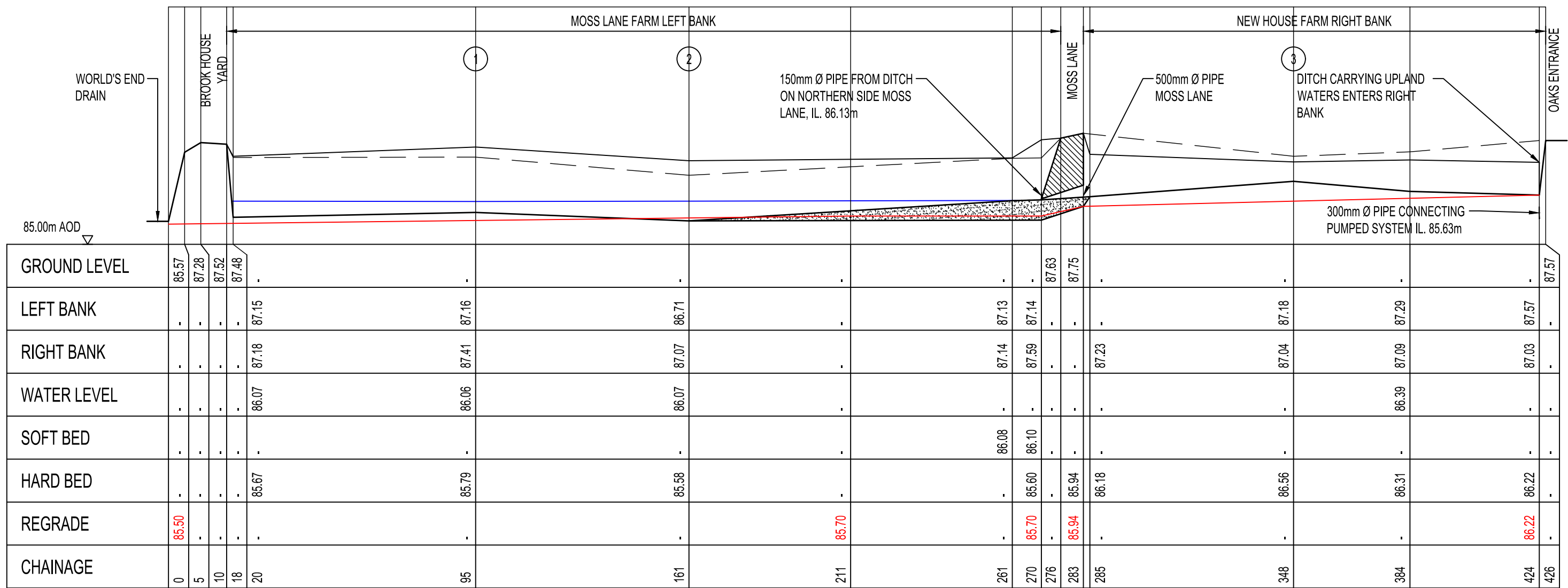
LONG SECTION (SCALE (H) 1:1250 (V) 1:100)
